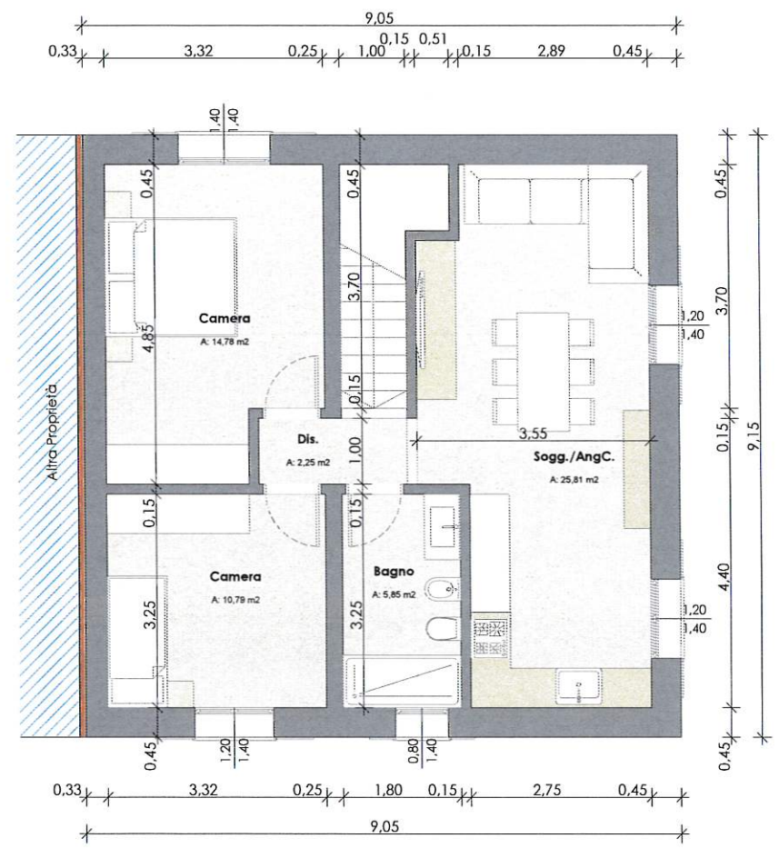
Piano Primo
